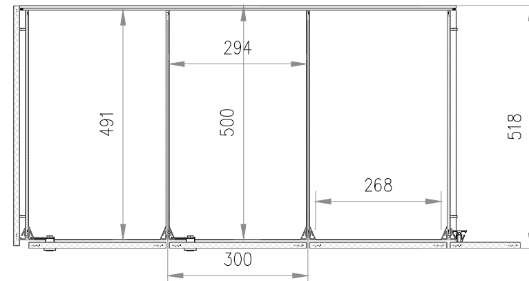
doorsnede bovenaanzicht
